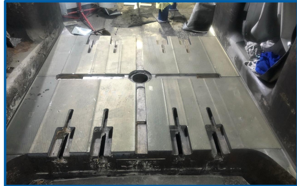
Pressentisch nach dem Laser-Pulver- Auftragschweißen
